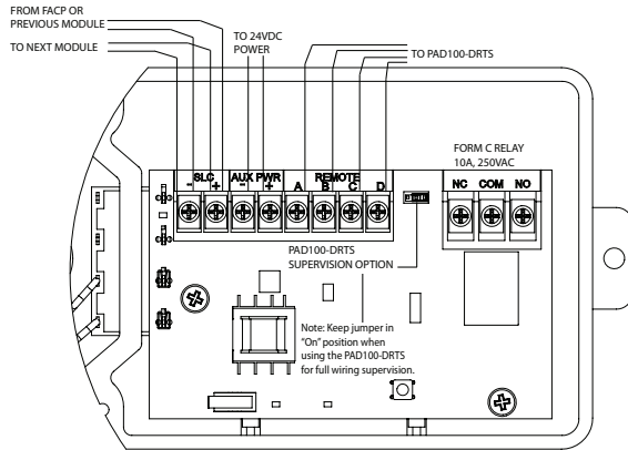
PAD100-DRTS Wiring
