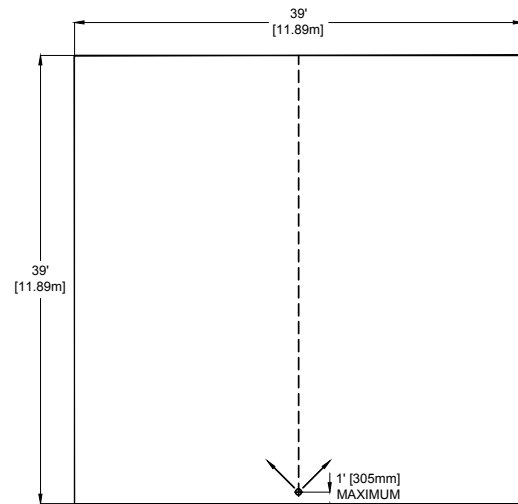
Configuración de boquilla lateral de 180° (6 orificios)
